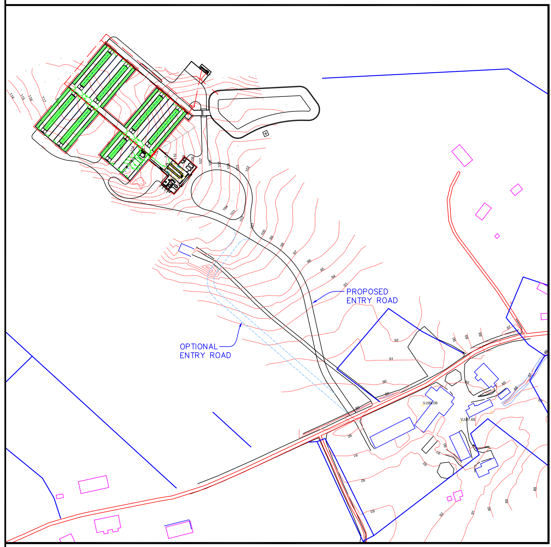
PLOT PLAN SCALE: 1:200
